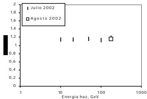
Figura 2. Valores medios del ratio pC/GeV para haces de e de diferentes energías. Agosto 2002.
