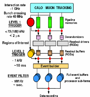
Figura 1. Sistema de adquisición de datos general del detector ATLAS con tres niveles de discriminación (triggers).
