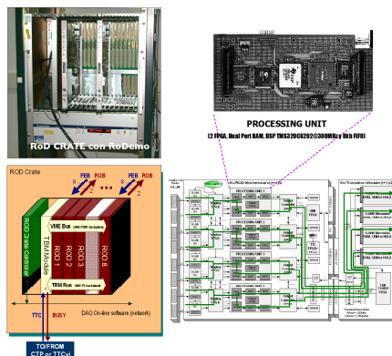
Figura 2. Sistema de lectura ROD organizado en cuatro particiones. La figura muestra una partición (1 ROD crate), la foto del prototipo RODdemo y un detalle de la unidad de proceso (PU) con DSP (4 por ROD motherboard)
