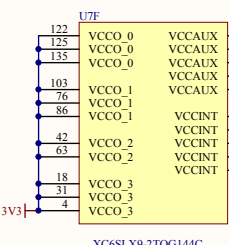
VCCAUX para JTAG interface VCCO_2 para linea memoria (3.3V)
