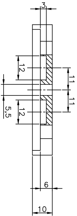
SECCION A-A
