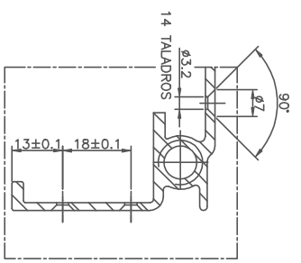
DETALLE B
